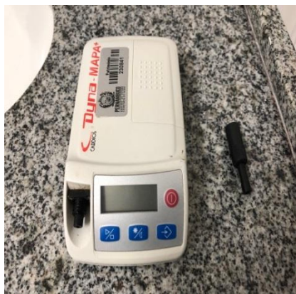
Imagem real do conector (peça preta) e equipamento (Gravador Dyna-Mapa+).
